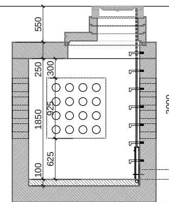
ŘEZ B-B
