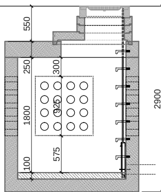
ŘEZ B-B
