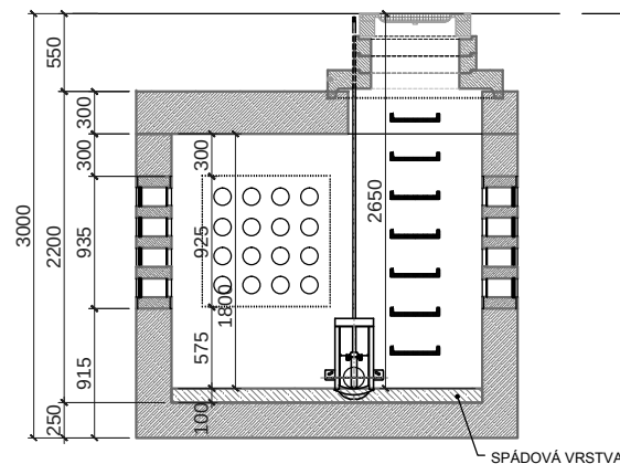
ŘEZ A-A
